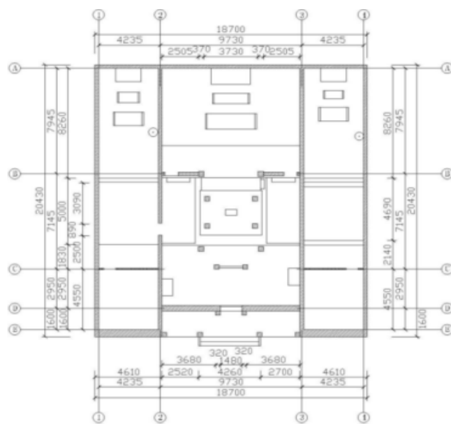
图3 淇澳岛文昌宫建筑平面图
